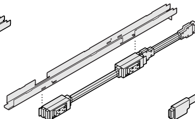
Powerkit Specifying ▶ Page B77
